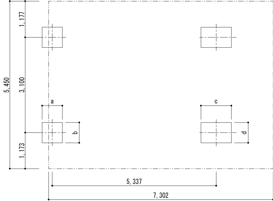
■ 基礎配置図
